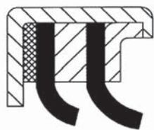
Tipo Lip seal D
