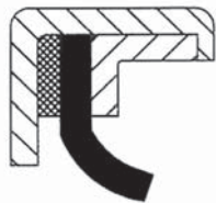
Tipo Lip seal S
